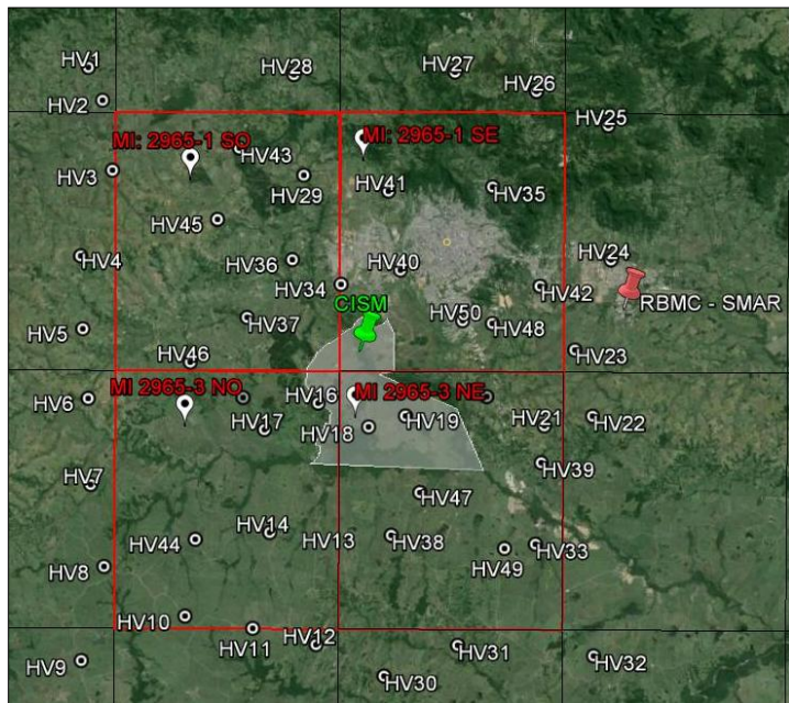
Distribuição dos Pontos de Apoio e de Controle no Entorno do CISM
